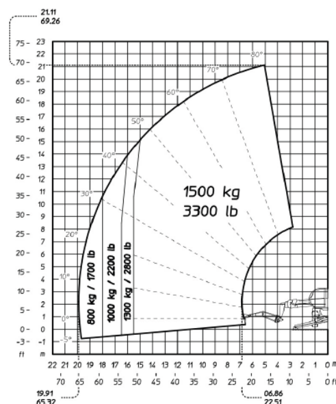
Drehung an abgesenkten Stützen mit 1500 kg Ausleger
