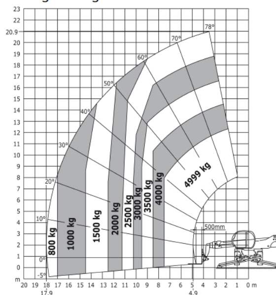
Drehung mit abgesenkten Stützen mit Gabeln
