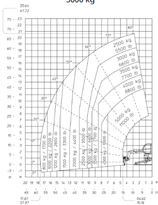
Drehung mit abgesenkten Stützen mit Seilwinde 5000 kg
